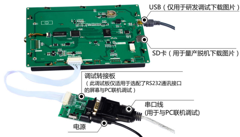
图 1-5 调试工具图
