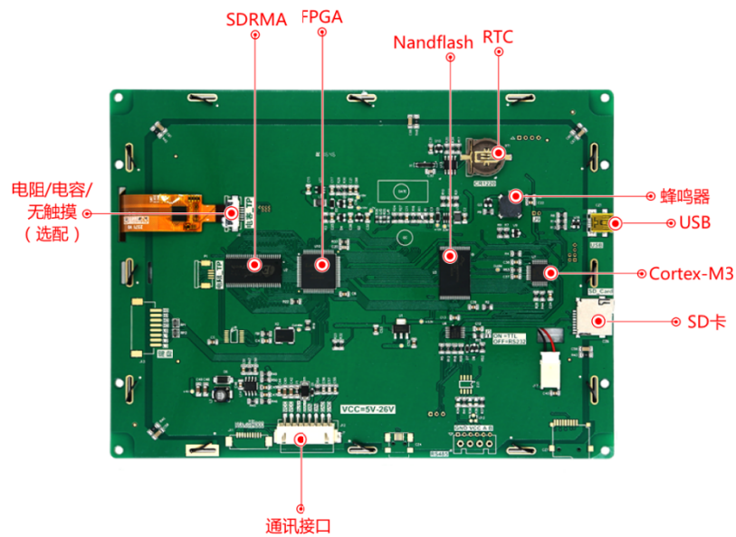
图 1-4 硬件配置图
